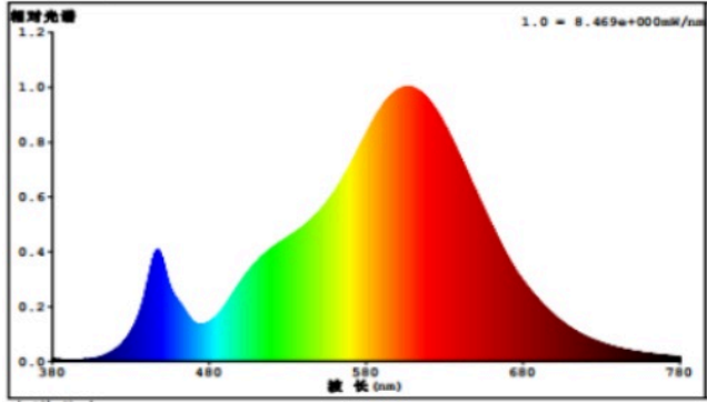
光谱参数
