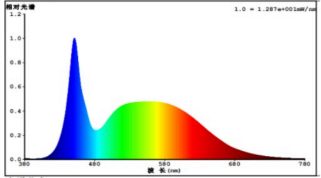
光谱参数
